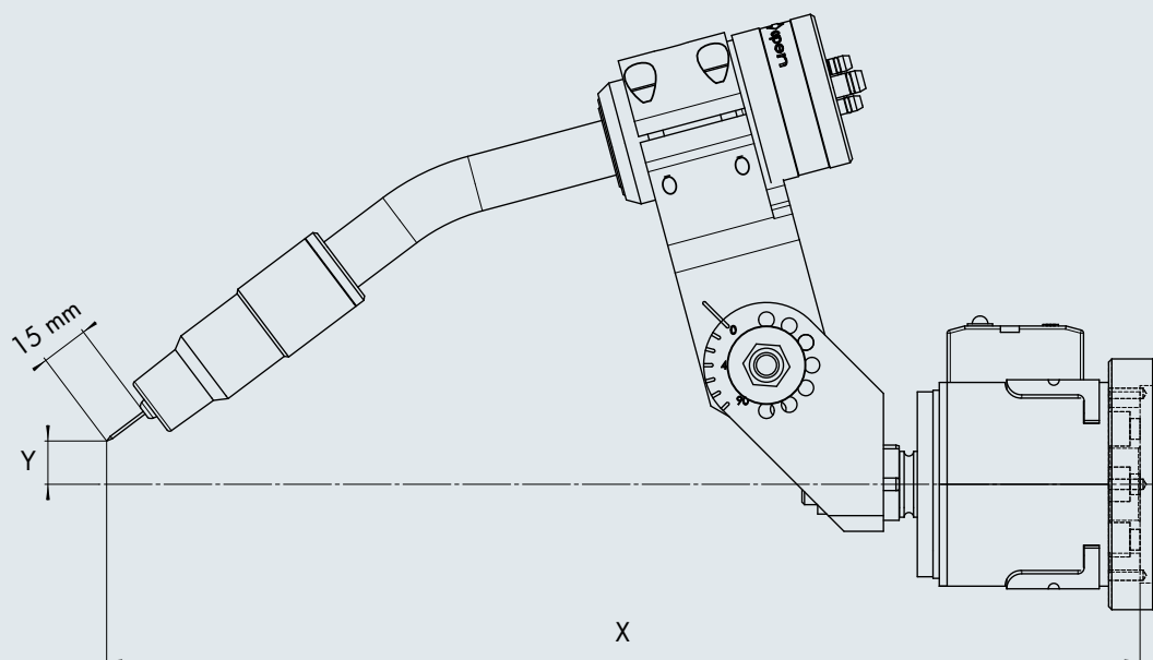
ROBO VTS z uchwytem mocującym regulowanym
